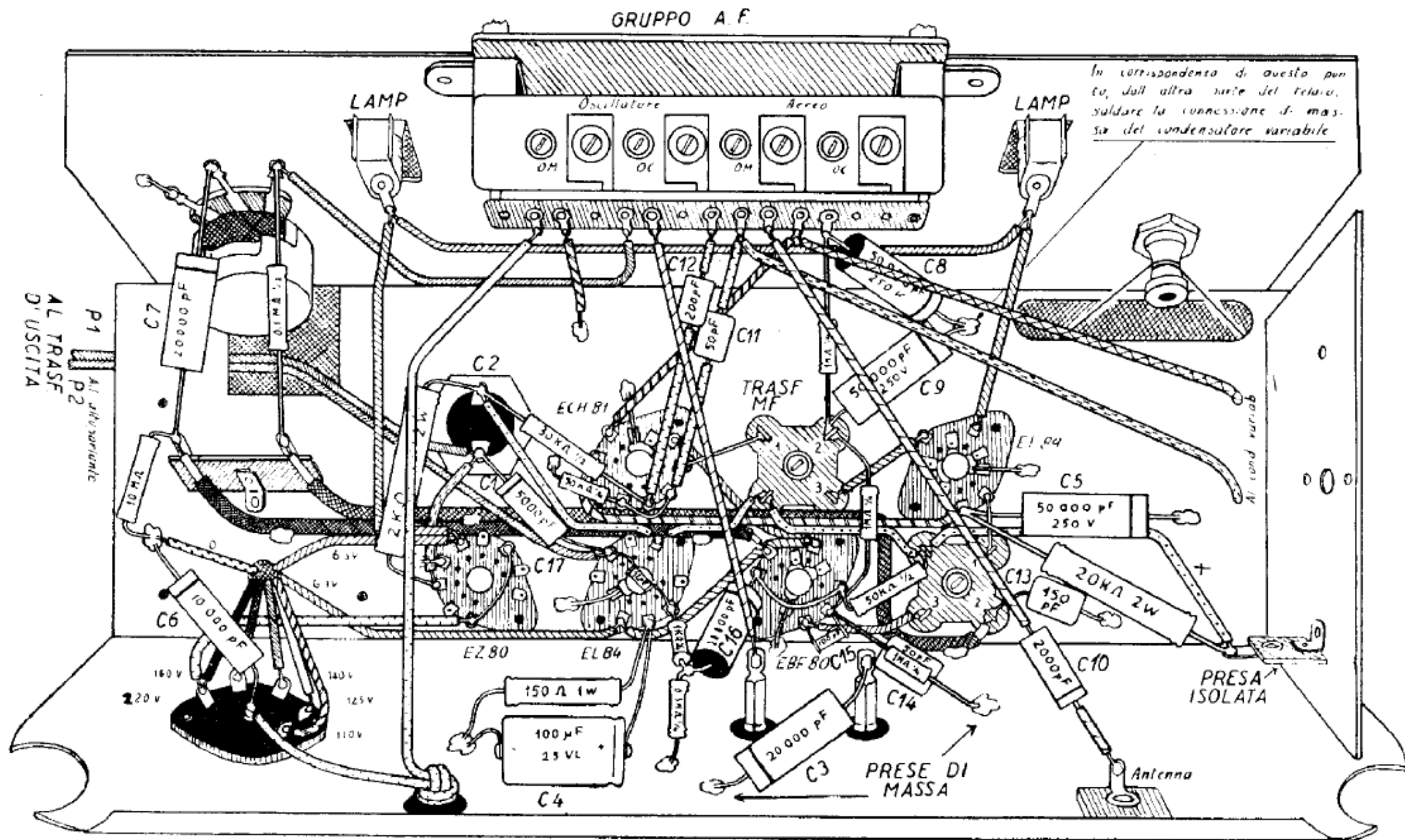
- Piano di montaggio dell'apparecchio « Modulina AM ».
